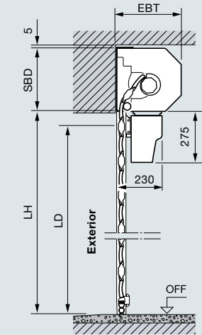
Campo de medidas para la puerta enrollable interior y exterior
