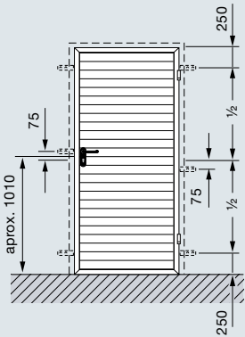
1 hoja sin anclaje inferior
