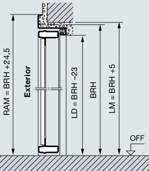
Anclaje exterior, apertura hacia el exterior
