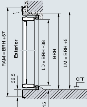
1 hoja con anclaje inferior
