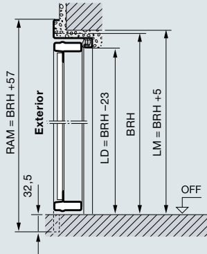
Anclaje interior, apertura hacia el interior
