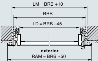
Anclaje exterior, apertura hacia el exterior
